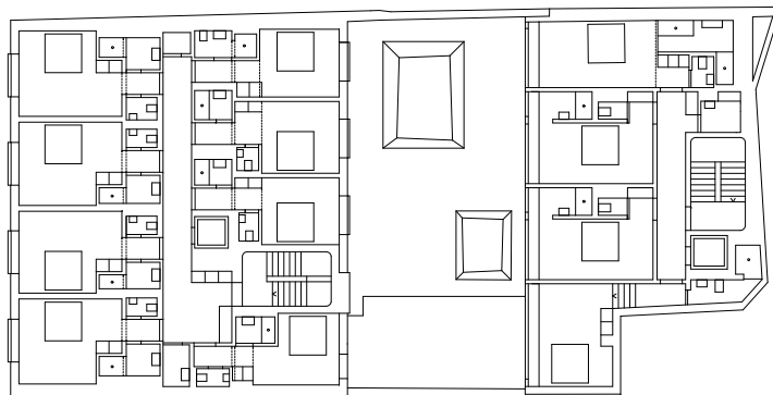
Grundriss 2 - 5. OG, Mst. 1:400
