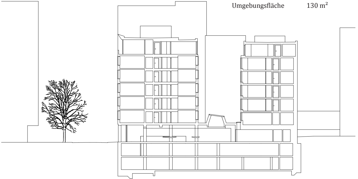
Schnitt, Mst. 1:400
