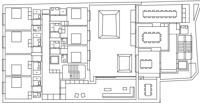
Grundriss 1. OG, Mst. 1:400
